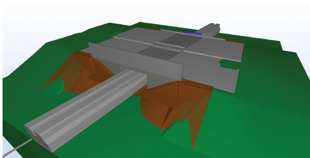
Abbildung 12: BIM-Pilotprojekt A99 Ersatzneubau BW 27/1 der Obersten Baubehörde im Bayerischen Ministerium des Innern, für Bau und Verkehr (Quelle: SSF-Ingenieure)
